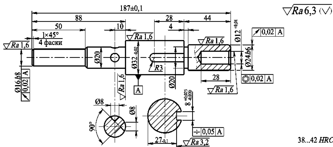
Рис. А 10. Вал промежуточный
